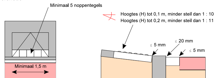
Bovenaanzicht
